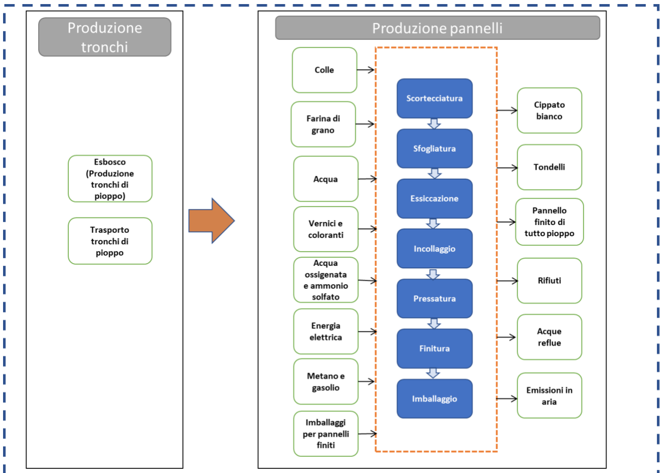
Figura 4. Confini del sistema della produzione del pannello in compensato di tutto pioppo.
