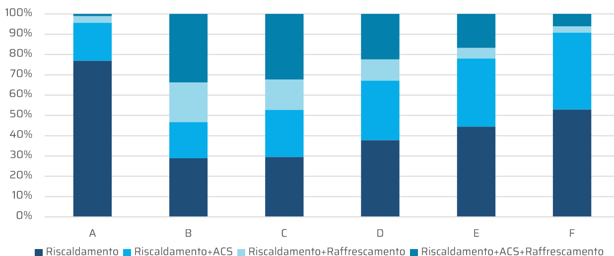
Figura 4.56 - SuperEcobonus al 31/12/2025. Servizi energetici gestiti dal sistema di BA, per zona climatica
