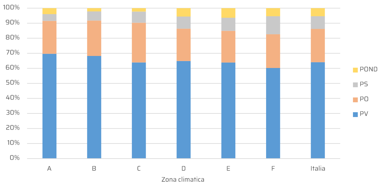
Figura 4.24 - Super Ecobonus al 31/12/2025. Distribuzione percentuale degli interventi di isolamento termico dell'involucro opaco, in termini di superficie, a livello nazionale e in ciascuna zona climatica
