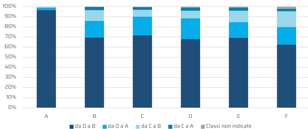
Figura 4.55 - SuperEcobonus al 31/12/2025. Variazioni di classe di automazione in ciascuna zona climatica
