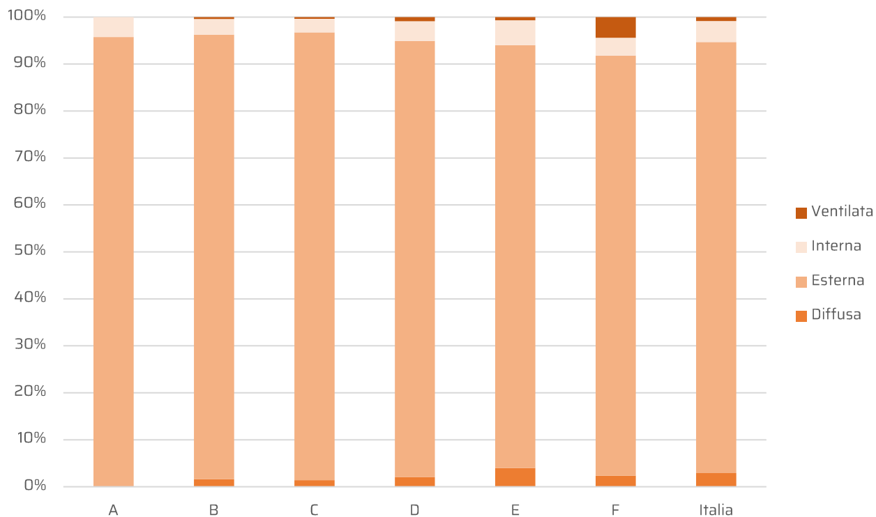
Figura 4.26 - SuperEcobonus al 31/12/2025. Distribuzione della superficie isolata di coperture disperdenti (PO) suddivisa per zona climatica e soluzione d'intervento
