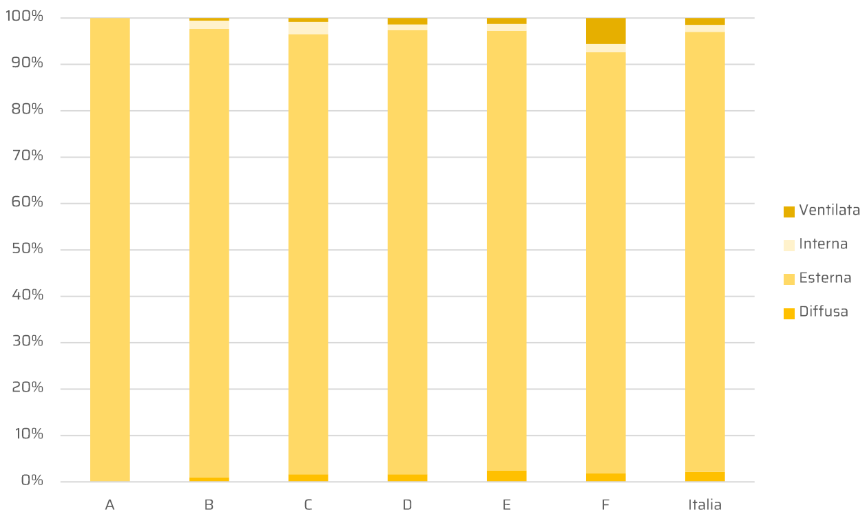
Figura 4.28 - SuperEcobonus al 31/12/2025. Distribuzione della superficie isolata di copertura non disperdente (POND) suddivisa per zona climatica e soluzione d'intervento
