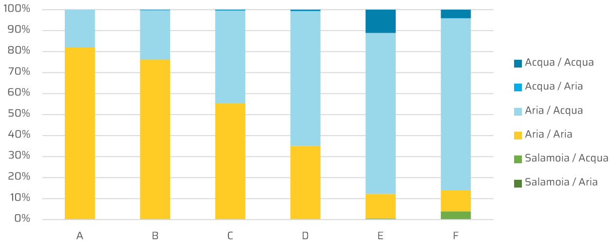
Figura 4.40 - SuperEcobonus al 31/12/2025. Distribuzione in ciascuna zona climatica delle pompe di calore a compressione di vapore elettriche rispetto alla potenza installata
