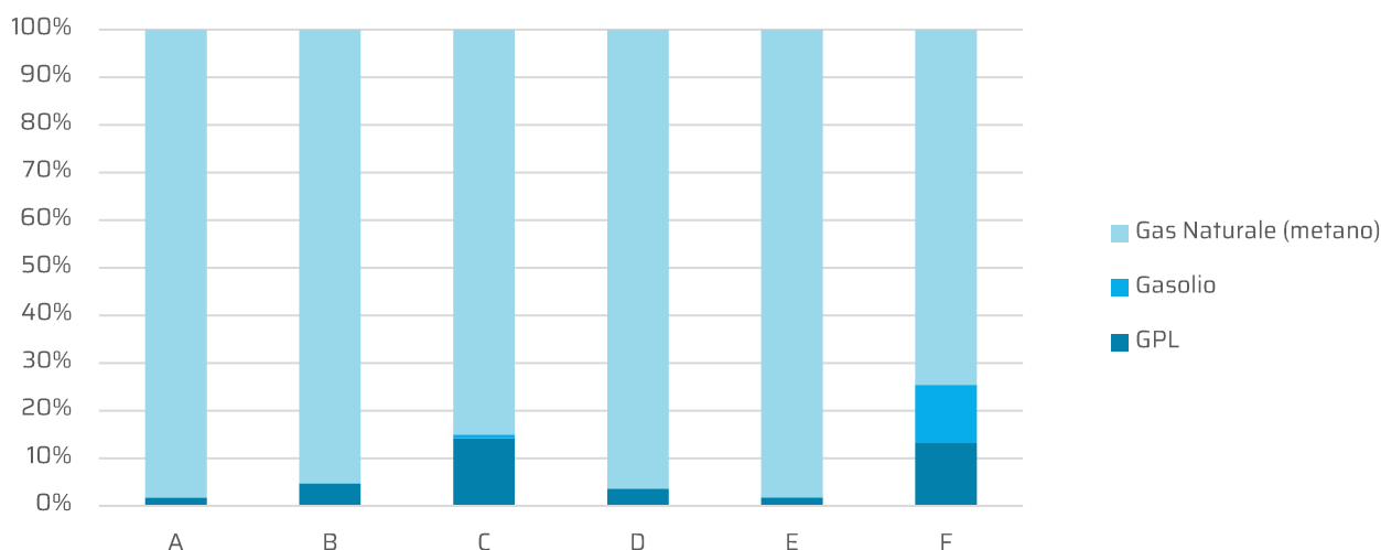
Figura 4.39 - SuperEcobonus al 31/12/2025. Distribuzione delle caldaie a condensazione rispetto al tipo di alimentazione, in funzione della potenza termica installata, per zona climatica
