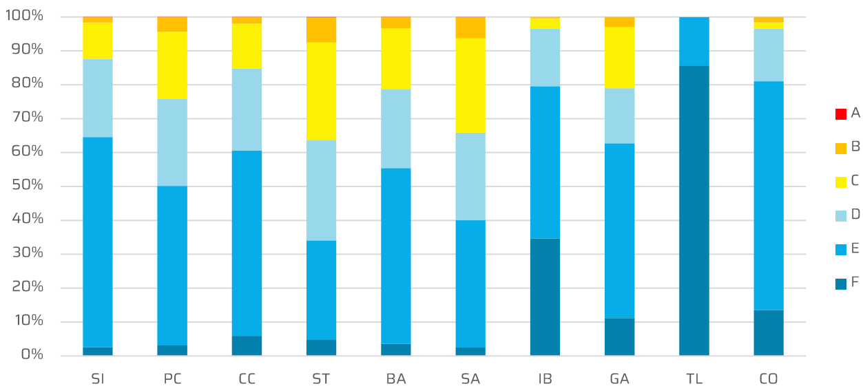
Figura 4.33 - SuperEcobonus al 31/12/2025. Distribuzione per zona climatica dei risparmi energetici connessi alle tecnologie adottate per il miglioramento degli impianti di climatizzazione invernale e a.c.s.
