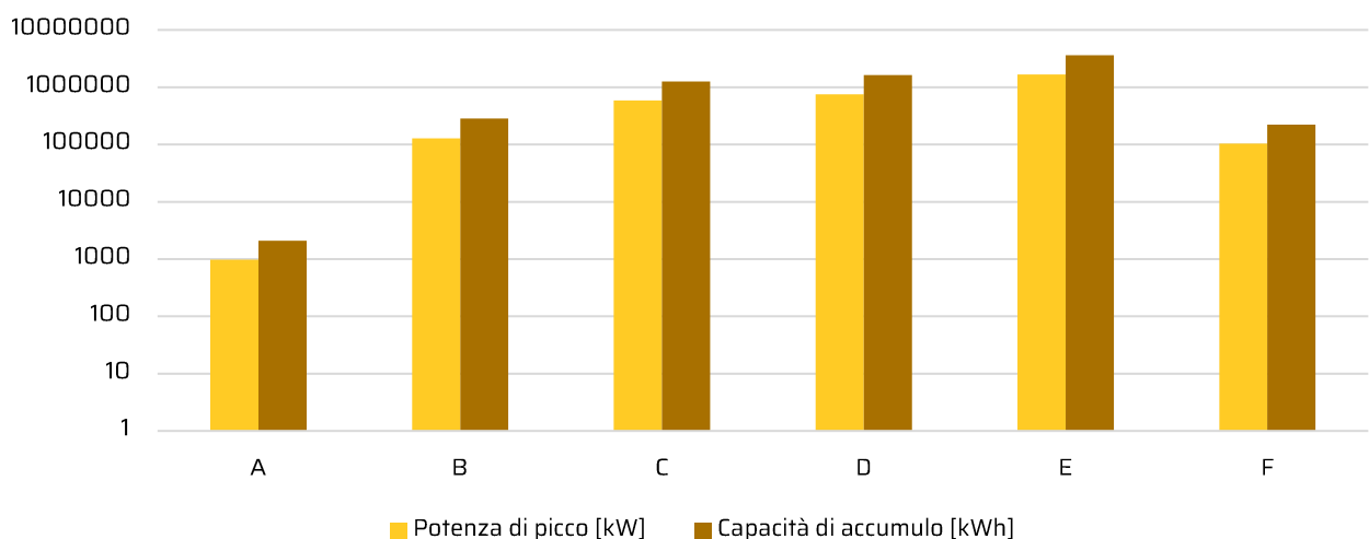
Figura 4.58 - SuperEcobonus al 31/12/2025. Potenza nominale d'impianto fotovoltaico e capacità di accumulo complessiva per zona climatica
